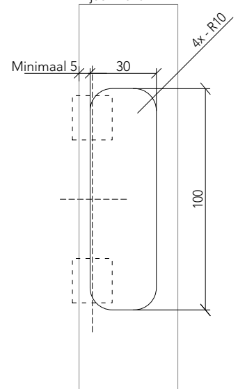
Inkrozing kozijn Zijaanzicht
